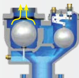
Evacuación de grandes cantidades de aire durante el llenado.
