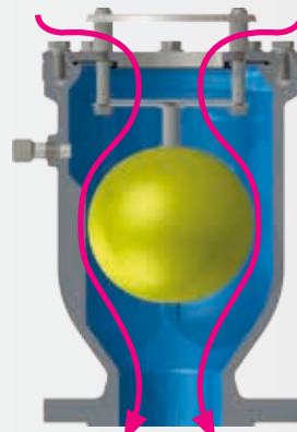
VACIADO DE LA TUBERÍA
