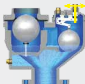
Purga de aire en carga.
