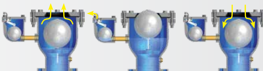
Evacuación de grandes cantidades de aire durante el llenado.
