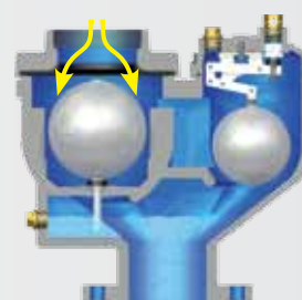
Admisión de grandes cantidades de aire durante el vaciado.
